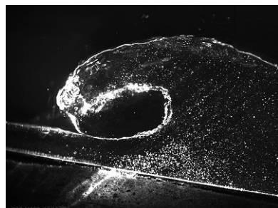
高速カメラで撮影した巻き波砕波
