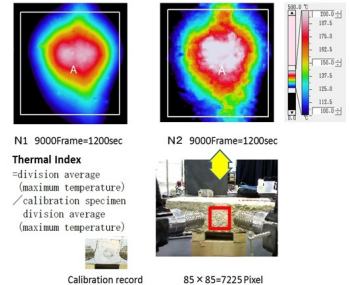
コンクリート表面品質のサーモグラフィ点検
