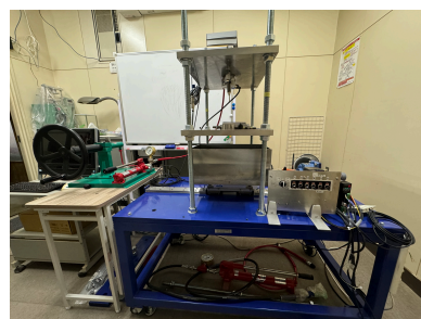
大型一面せん断試験機
