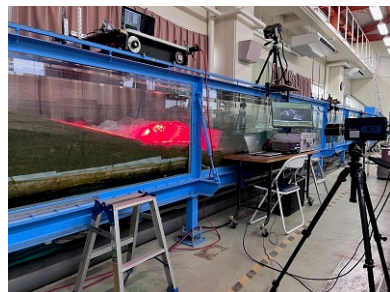
高速カメラと画像解析システム
