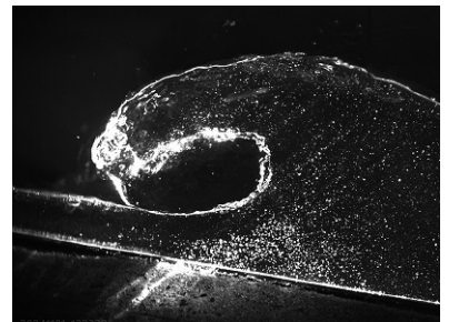
高速カメラで撮影した巻き波砕波
