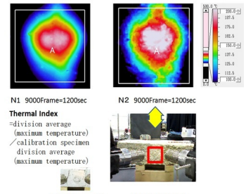
コンクリート表面品質のサーモグラフィ点検
