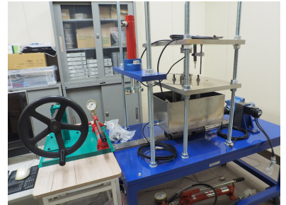
大型一面せん断試験機
