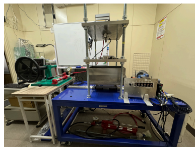
大型一面せん断試験機
