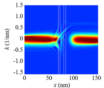
共鳴トンネルダイオードの 共鳴トンネル時のウィグナー関数
